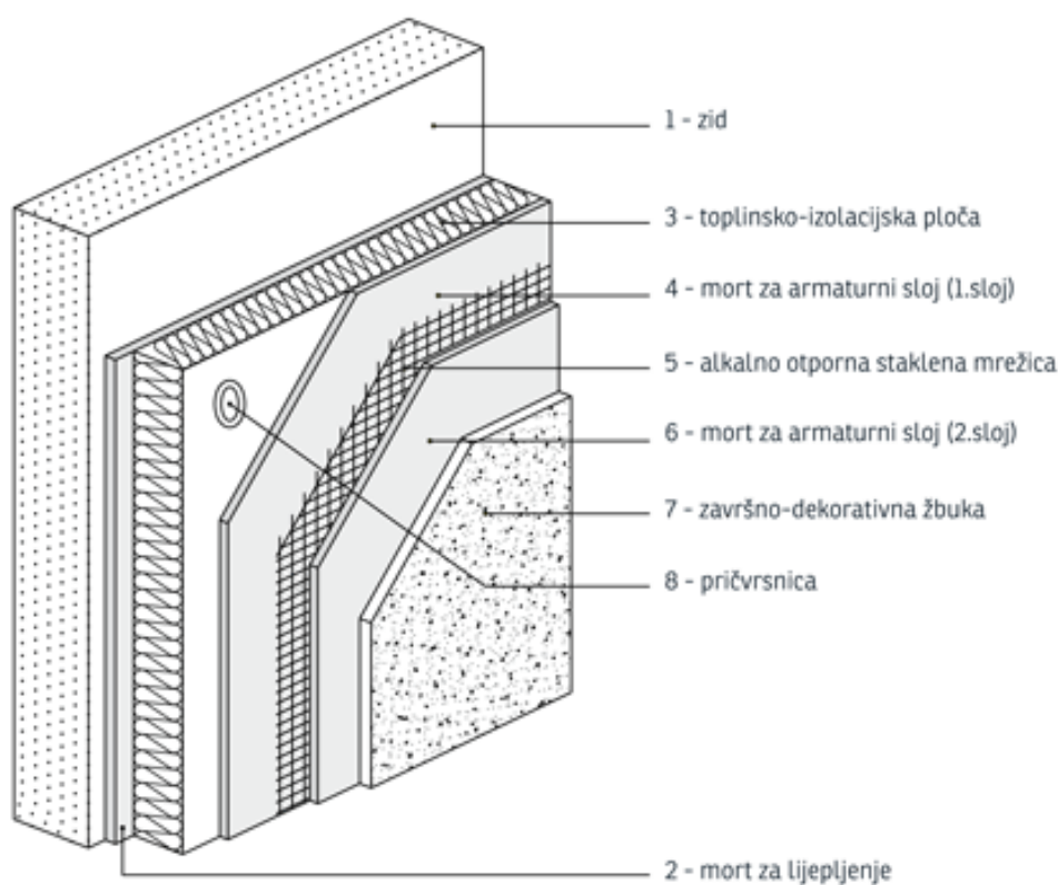
Slika 1 Prikaz povezanog toplinsko-fasadnog sustava
